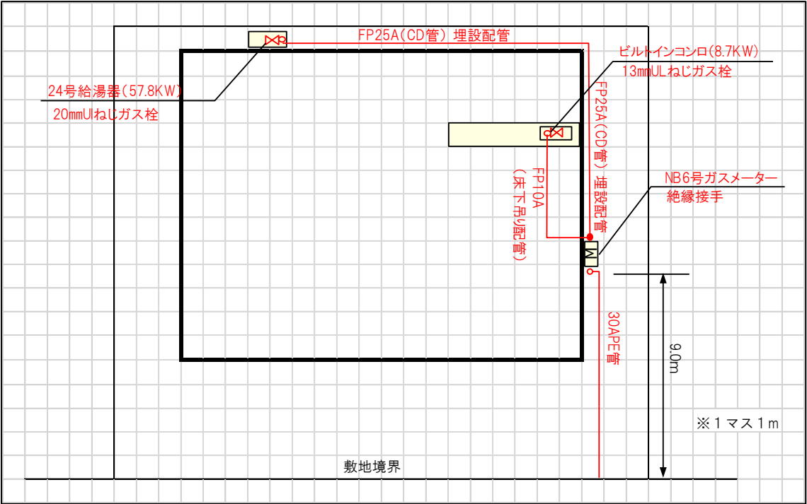
<内管工事の標準モデル図>
